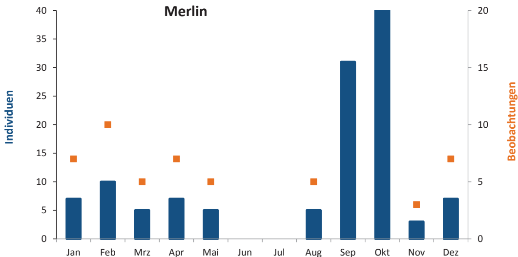
Abb. 5: Auftreten des Merlins Falco columbarius in Mecklenburg-Vorpommern 2014 (123 Beob., 136 Ind.; Quelle: ornitho.de und oamv.de). – Fig. 5: Occurrence of the Merlin in Mecklenburg-Western Pomerania in 2014 (observations n=123, individuals n=136; data from www.ornitho.de and www.oamv.de).
