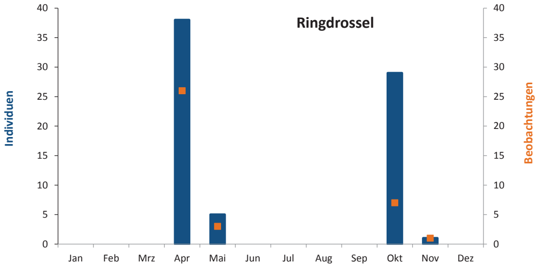
Abb. 12: Auftreten der Ringdrossel Turdus torquatus in Mecklenburg-Vorpommern 2014 (37 Beob., 73 Ind.; Quelle: ornitho.de und oamv.de). – Fig. 12: Occurrence of the Ring Ouzel in Mecklenburg-Western Pomerania in 2014 (observations n=37, individuals n=73; data from www.ornitho.de and www.oamv.de).
