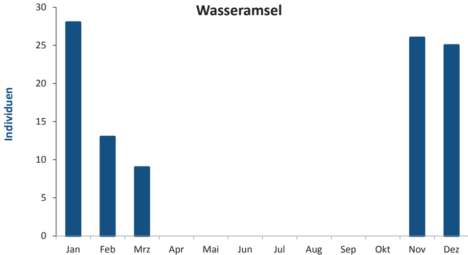
Abb. 11: Auftreten der Wasseramsel Cinclus cinclus in Mecklenburg-Vorpommern 2014 (101 Ind., an einigen Standorten hielten sich Vögel über einen längeren Zeitraum auf, daher können diese mehrfach erfasst worden sein; Quelle: ornitho.de und oamv.de). – Fig. 11: Occurrence of the White-throated Dipper in Mecklenburg-Western Pomerania in 2014 (totals may include double-countings, especially in case of occurrence for several days; individuals n=101; data from www.ornitho.de and www.oamv.de).
